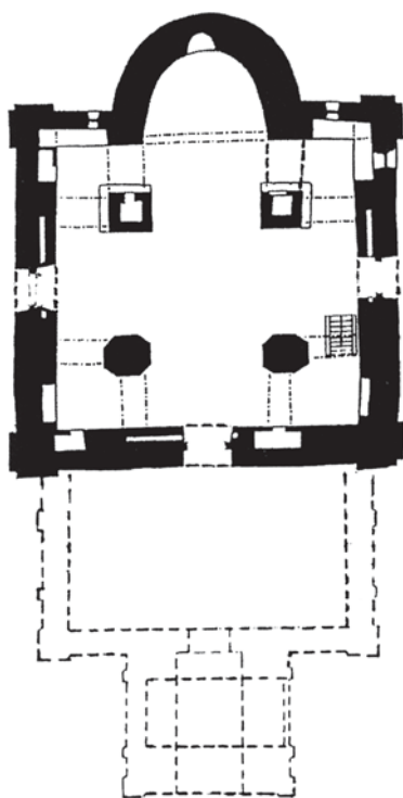
Рис. 2. План церкви на Липне
